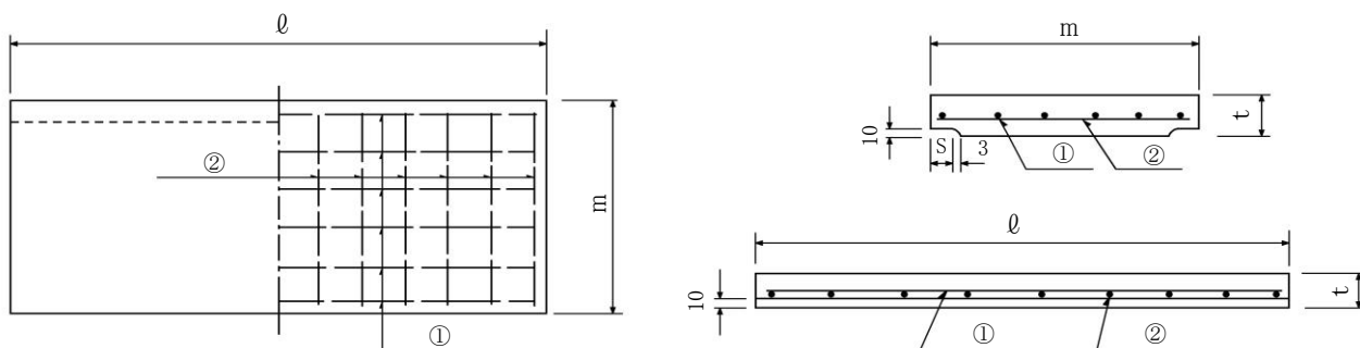
■ I 形の寸法及び配筋表 T-14
